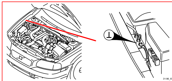
31/96 接地，右側麥弗森懸架
