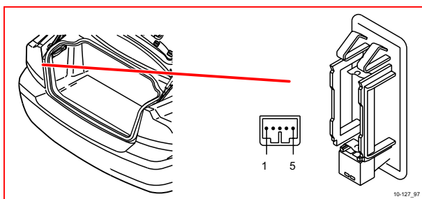
10/127 行李廂左側照明燈
