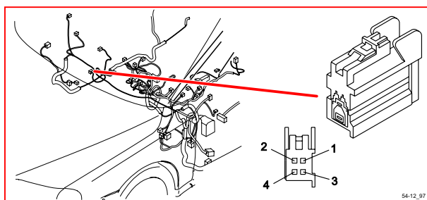
54/12 接頭
