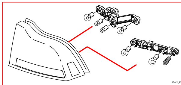
10/42 右後運行燈 / 駐車燈
