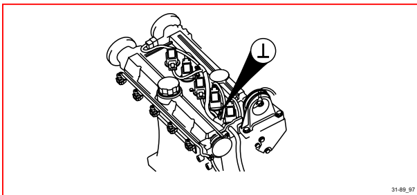
31/89 接地，引擎點火線圈組 2
