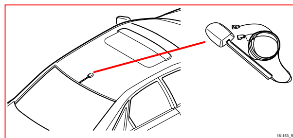
16/153 衛星收音機天線
