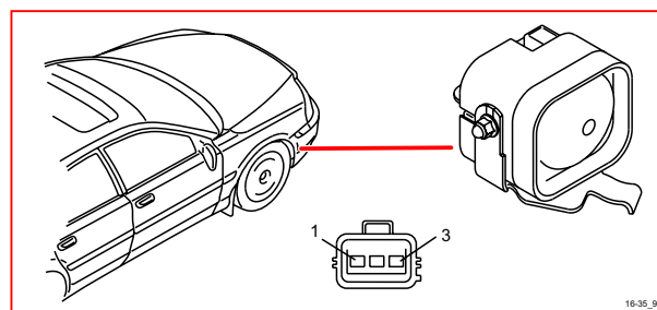
16/35 警笛控制模組 (SCM)
