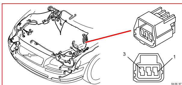
54/56 接頭
