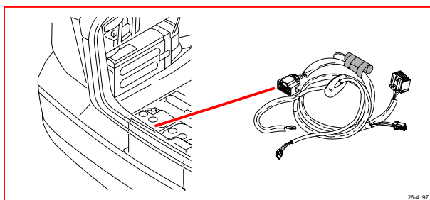
26/4 整流器，方向指示燈與煞車燈，美國
