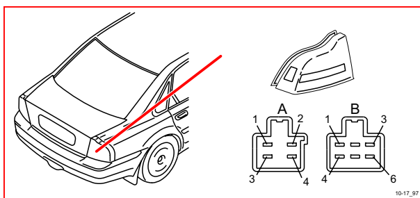
10/17 右後燈殼體
