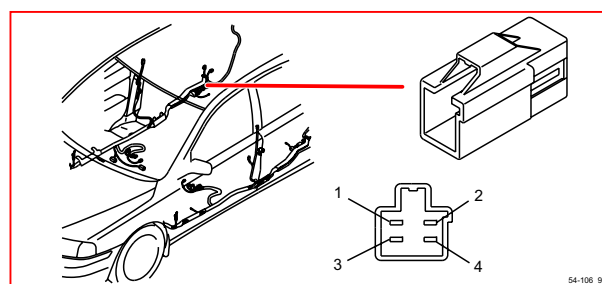
54/106 接頭
