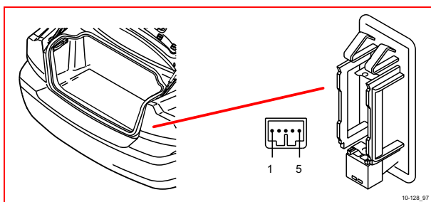
10/128 行李廂右側照明燈
