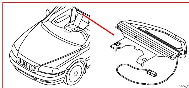
16/64 行動電話天線
