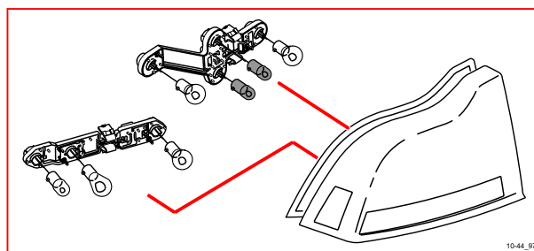
10/44 右尾燈 1
