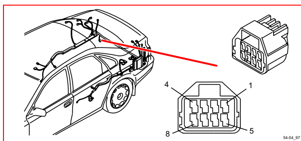
54/54 接頭
