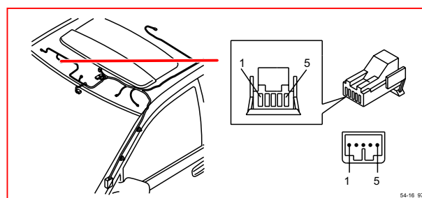
54/16 接頭
