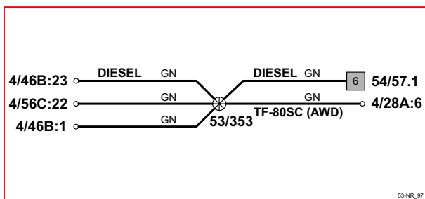
53/ 編號 分線點
