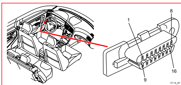
17/13 數據連線接頭
