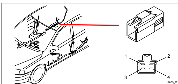
54/35 接頭
