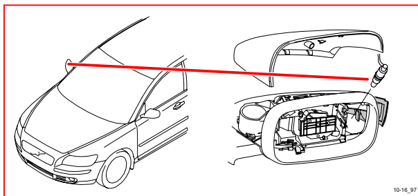
10/16 右側方向指示燈後視鏡
