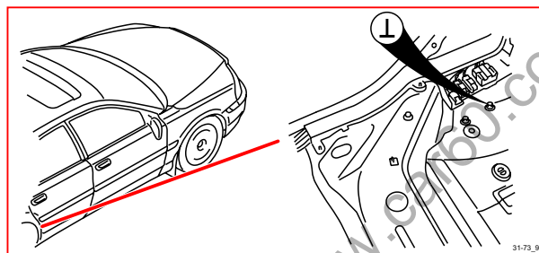
31/73 接地，右後座升降器
