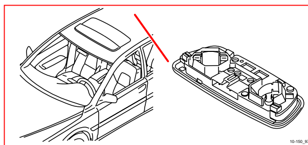
10/150 後閱讀燈
