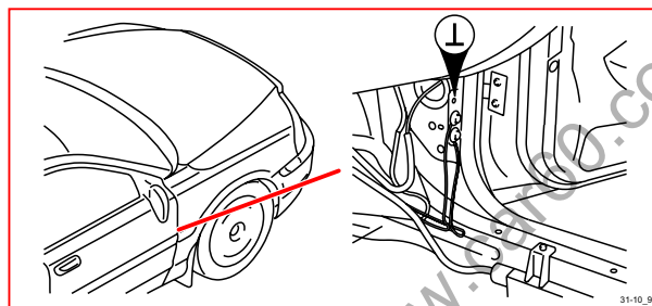
31/10 接地，A 柱右側
