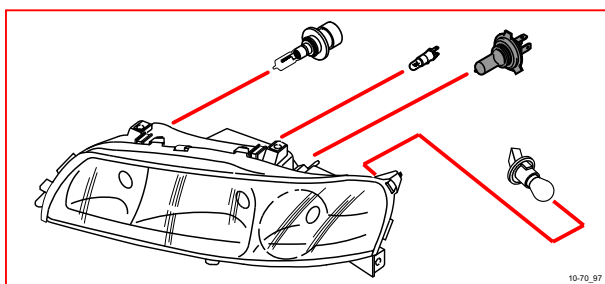
10/70 左近光燈
