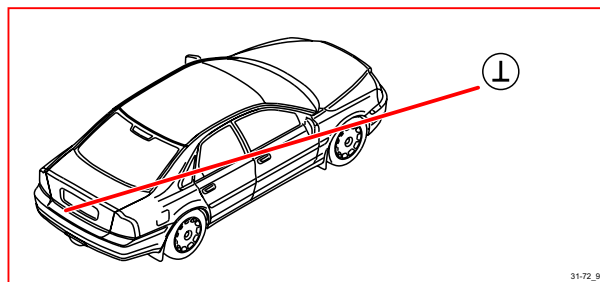
31/72 接地，行李廂
