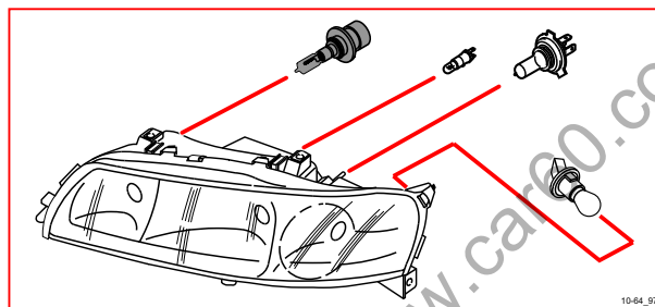
10/64 右遠光燈
