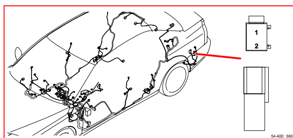
54/40D 接頭
