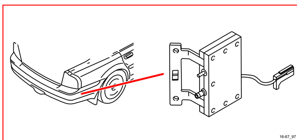
16/67 保險杠天線放大器
