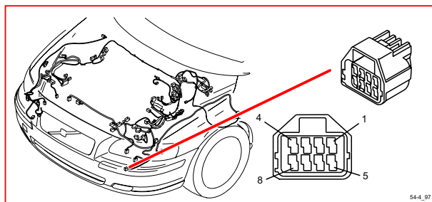
54/4 接頭
