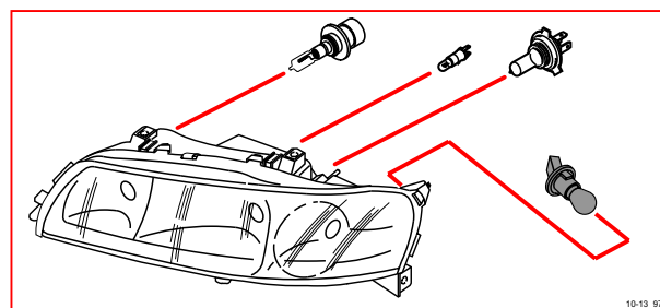
10/13 左前方向指示燈
