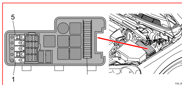
11 A/ 編號 引擎室保險絲盒內之主保險絲
