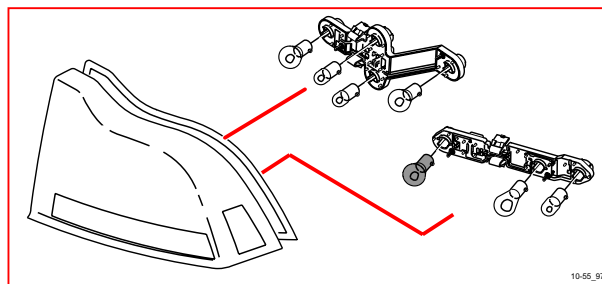
10/55 左倒車燈
