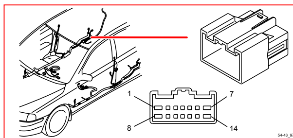
54/43 接頭
