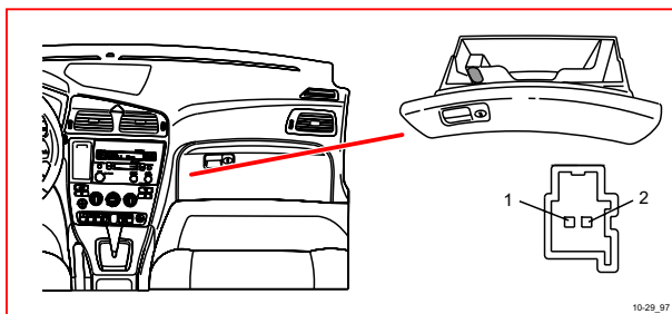
10/29 手套箱燈
