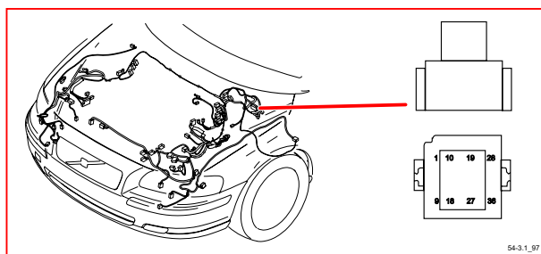
54/3.1 接頭
