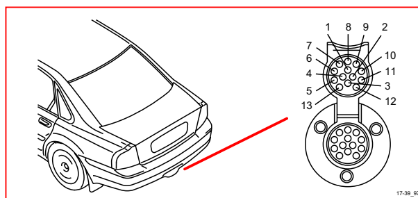
17/39 13 腳插座，拖車電纜線束
