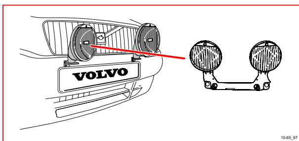
10/65 右前輔助燈
