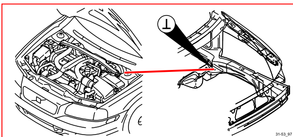
31/53 接地，橫向間壁
