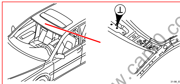
31/98 接地，擋風玻璃上橫梁
