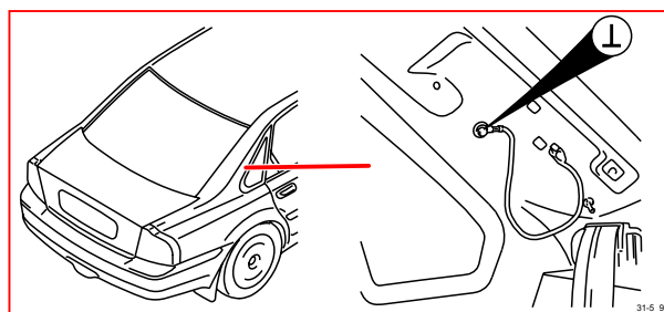
31/5 接地，右 D 柱
