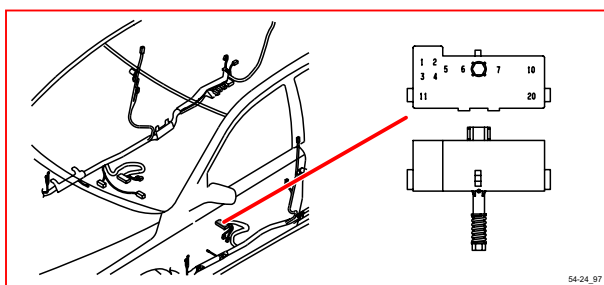
54/24 接頭
