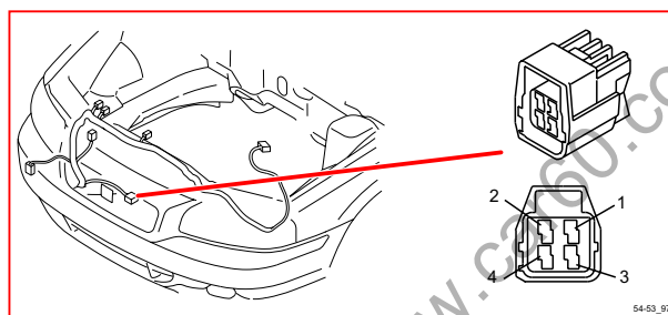
54/53 接頭
