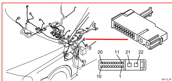
54/13 接頭
