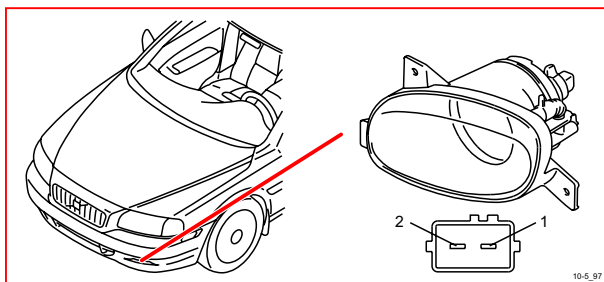
10/5 左前霧燈
