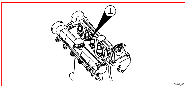
31/88 接地，引擎點火線圈組 1
