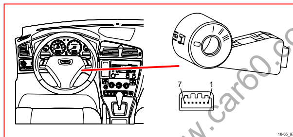
16/65 天線環 / 點火開關照明
