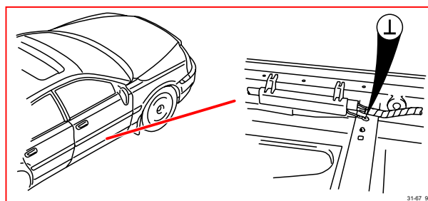
31/67 接地，前座椅升降機，右側
