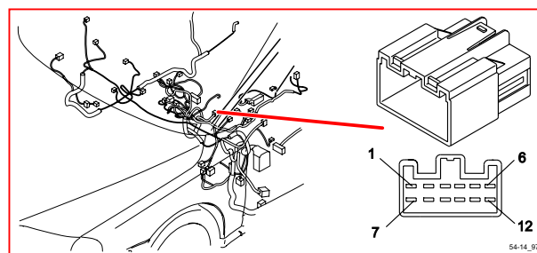
54/14 接頭
