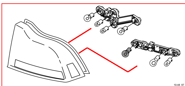
10/48 右倒車燈
