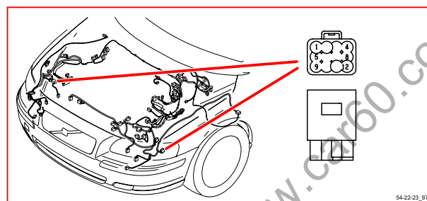
54/22-23 接頭
