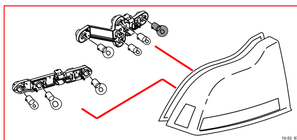
10/53 左後霧燈
