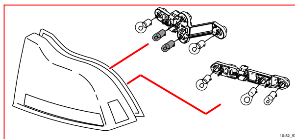
10/52 左後燈 2
