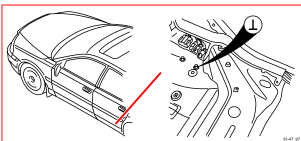
31/47 接地，右後座升降器
