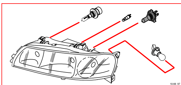
10/66 右近光燈
