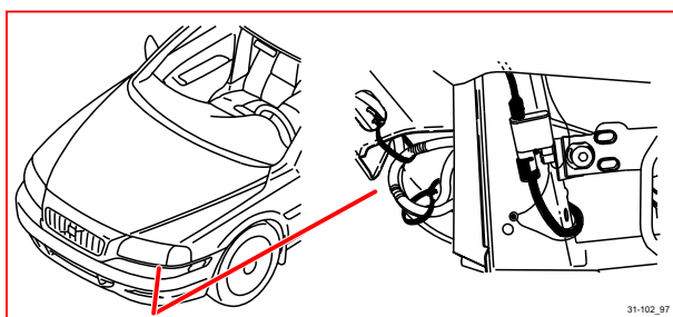
31/102 接地，前構件
