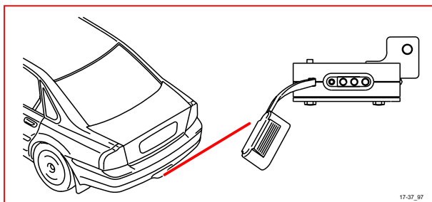
17/37 4 腳插座，拖車電纜線束
