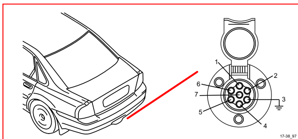
17/38 7 腳插座，拖車電纜線束
