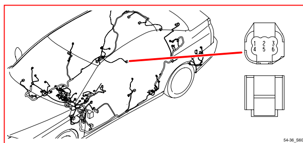
54/36 接頭
