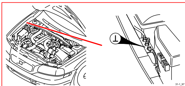
31/1 接地，右側麥弗森懸架
