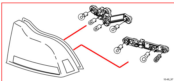
10/49 左後運行燈 / 駐車燈
