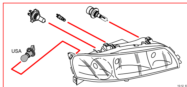
10/12 右前運行燈 / 駐車燈
