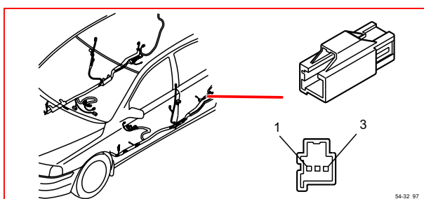
54/32 接頭
