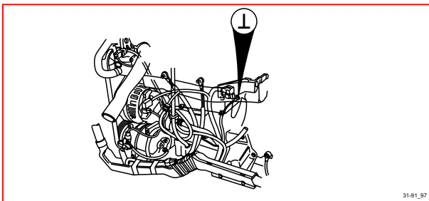
31/91 接地，引擎
