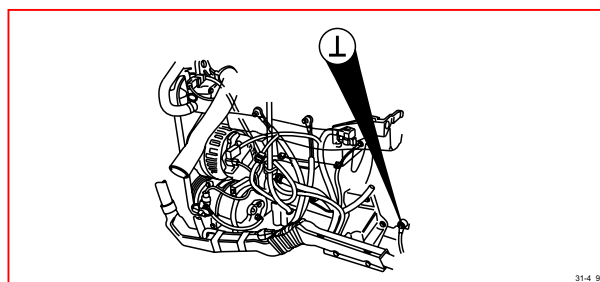
31/4 接地，引擎
