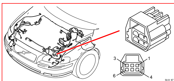
54/9 接頭
