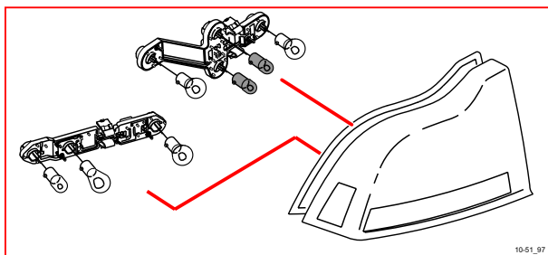
10/51 左後燈 1
