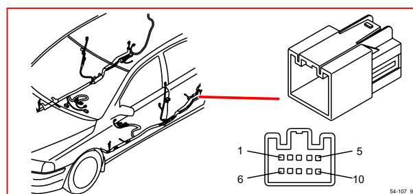
54/107 接頭
