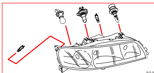
10/73 右前側運行燈
