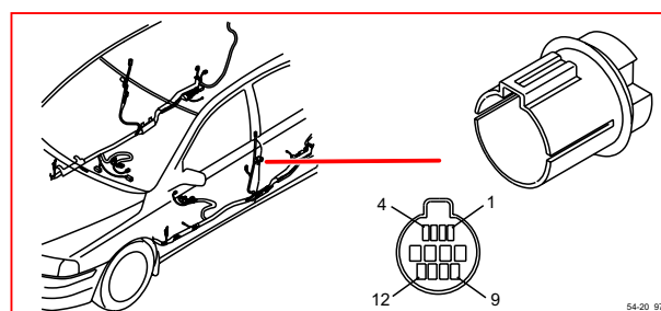
54/20 接頭
