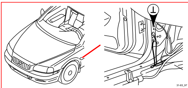
31/83 接地，左側 A 柱
