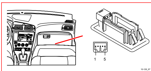
10/126 右前車門禮貌燈
