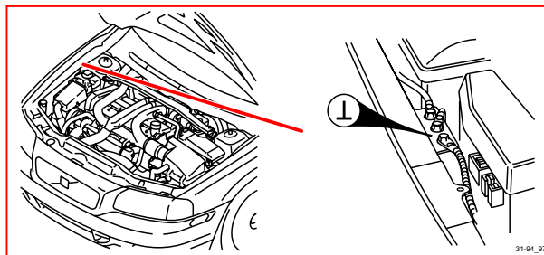
31/94 接地，右側麥弗森懸架
