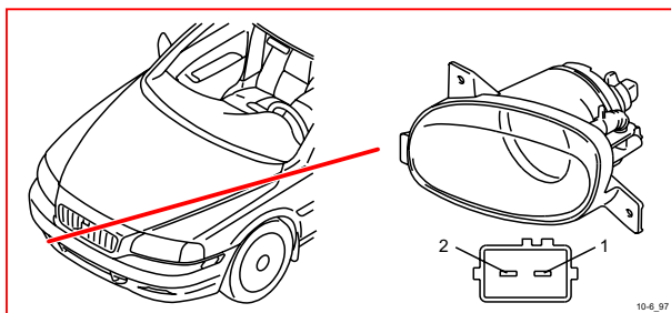
10/6 右前霧燈
