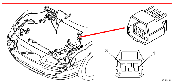
54/55 接頭
