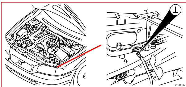
31/44 接地，引擎室左下部橫梁
