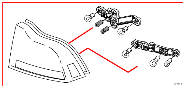
10/45 右尾燈 2
