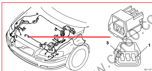
54/7 接頭
