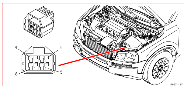
54/57.1 接頭
