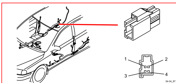
54/34 接頭
