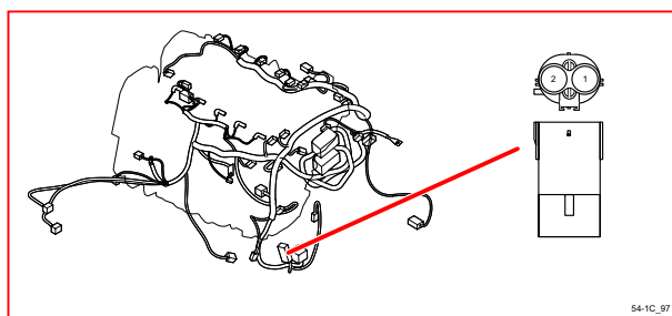
54/1C 接頭
