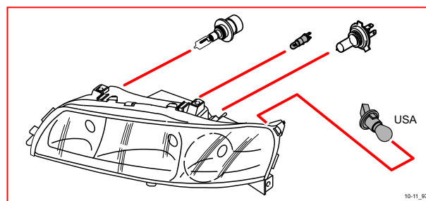
10/11 左前運行燈 / 駐車燈
