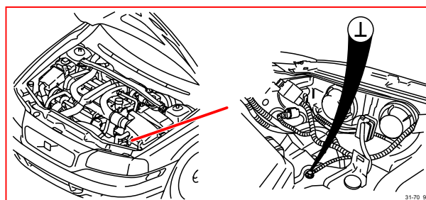
31/70 接地，引擎室左下部橫梁
