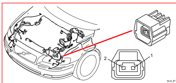
54/8 接頭
