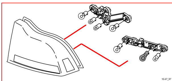
10/47 右後方向指示燈
