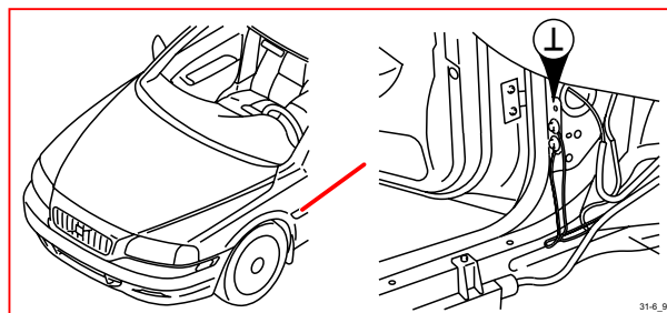
31/6 接地，駕駛員側 A 柱
