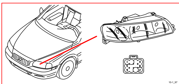
10/1 左前燈殼體
