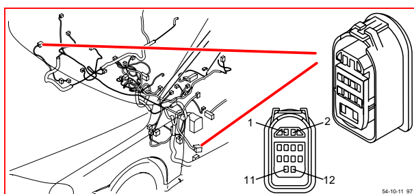
54/10-11 接頭
