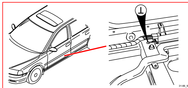
31/66 接地，前座椅升降機，左側
